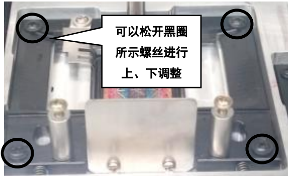
图 8.13 调整喷头机械位置
