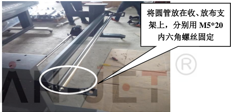
图 1.13 圆管安装示意图 (三)
