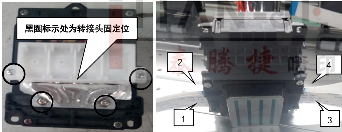
图 5.2 打印机喷头
